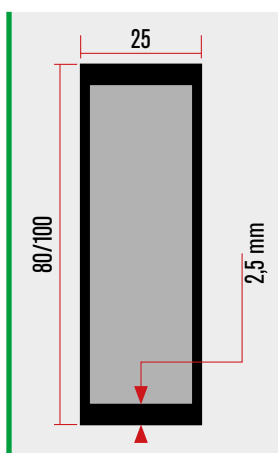
Profili a sezione rinforzata 2,5 mm. Sides with 2.5 mm reinforced section.
